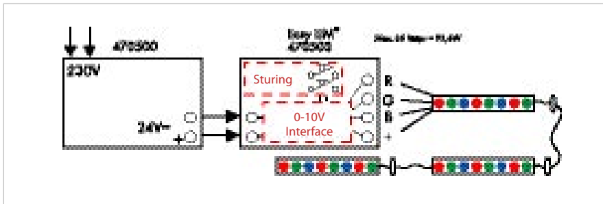
Aansluitschema met Easy LIM ® en netvoeding
