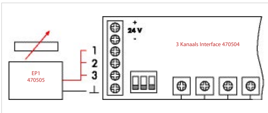
Aansluitschema voor 3 Kanaals interface met EP1
