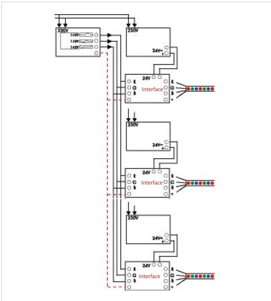
Aansluitschema van parallelschakeling bij grote vermogens.
